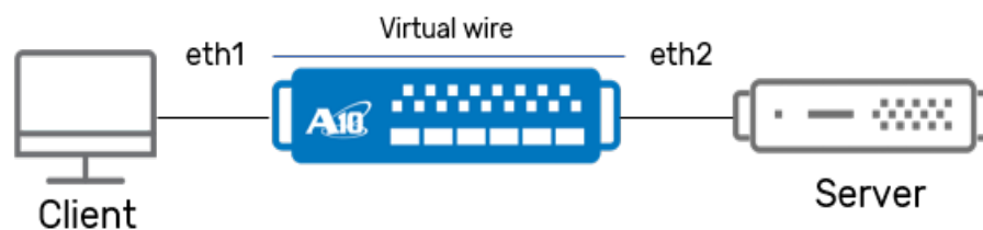
Figure 6 : Virtual Wire - Endpoints: E1 and E2
